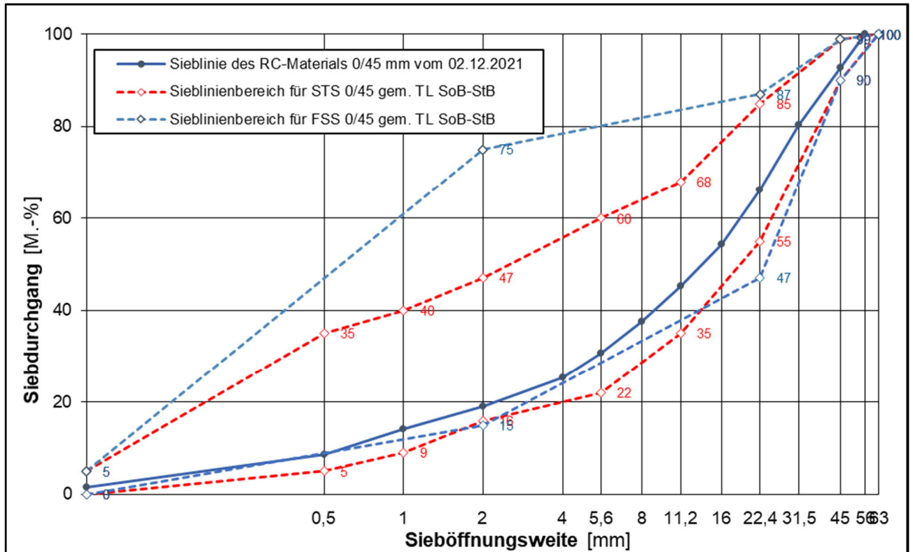
Korngrößenverteilung des untersuchten RC-Materials 0/45 mit Sieblinienbereich für Schottertragschichten 0/45 mm gemäß TL SoB-StB /8/
