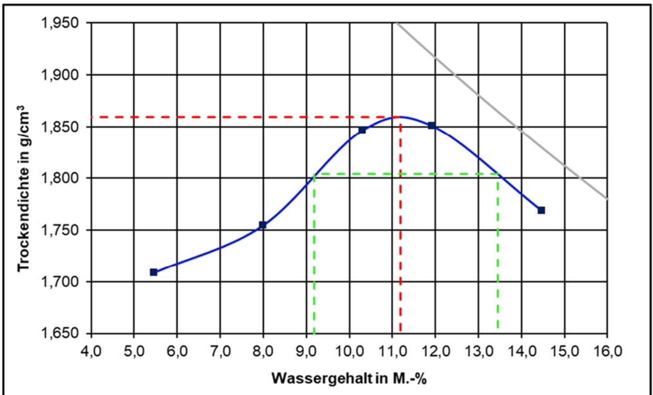
Proctorkurve des untersuchten RC-Materials 0/45 (aus Prüfbericht F 22/01/0041 – I/2022)
