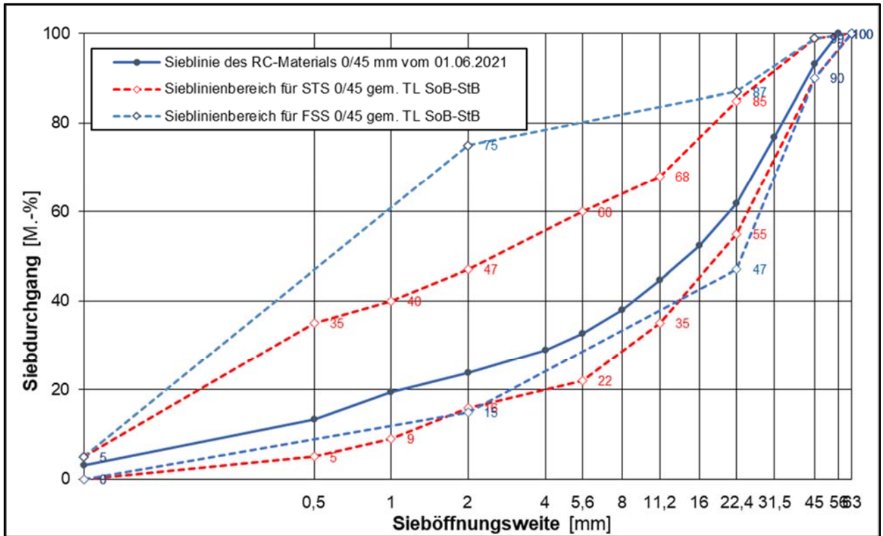
Korngrößenverteilung des untersuchten RC-Materials 0/45 mm mit Sieblinienbereich für Schottertragschichten 0/45 mm gemäß TL SoB-StB /8/
