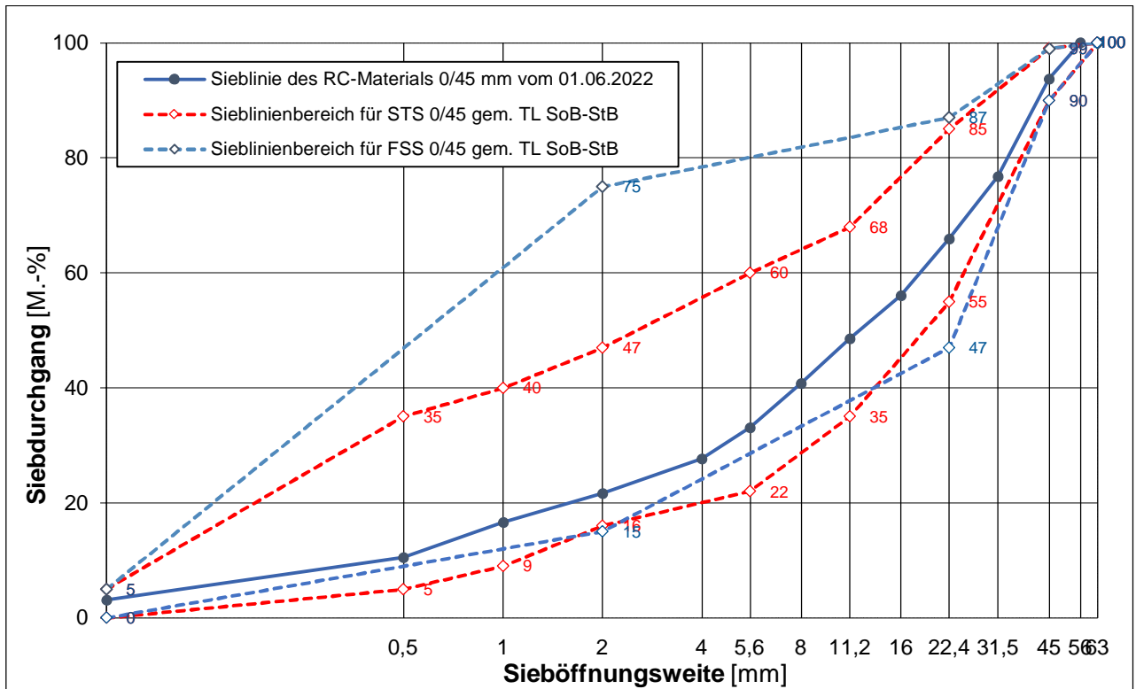
Korngrößenverteilung des untersuchten RC-Materials 0/45 mit Sieblinienbereich für Schottertrag- und Frostschutzschichten 0/45 mm gemäß TL SoB-StB /8/
