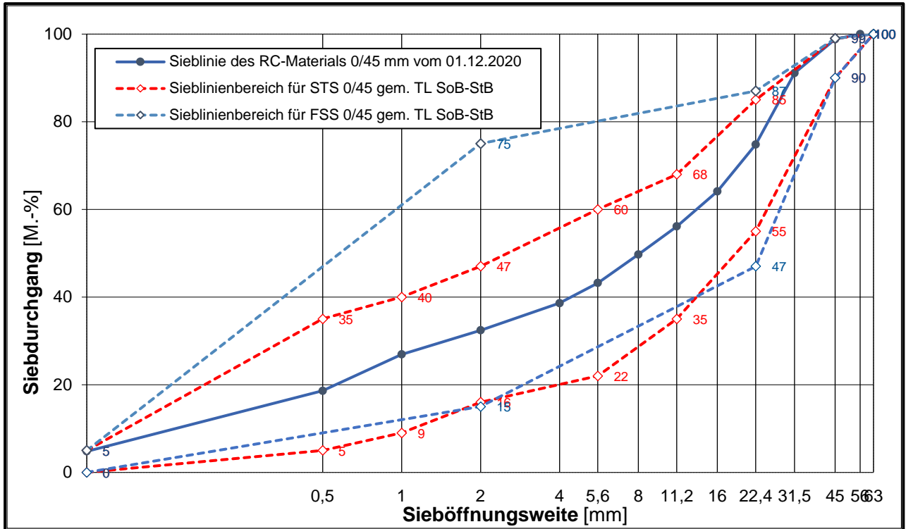
Korngrößenverteilung des untersuchten RC-Materials 0/45 mit Sieblinienbereich für Schottertragschichten 0/45 mm gemäß TL SoB-StB 7/
