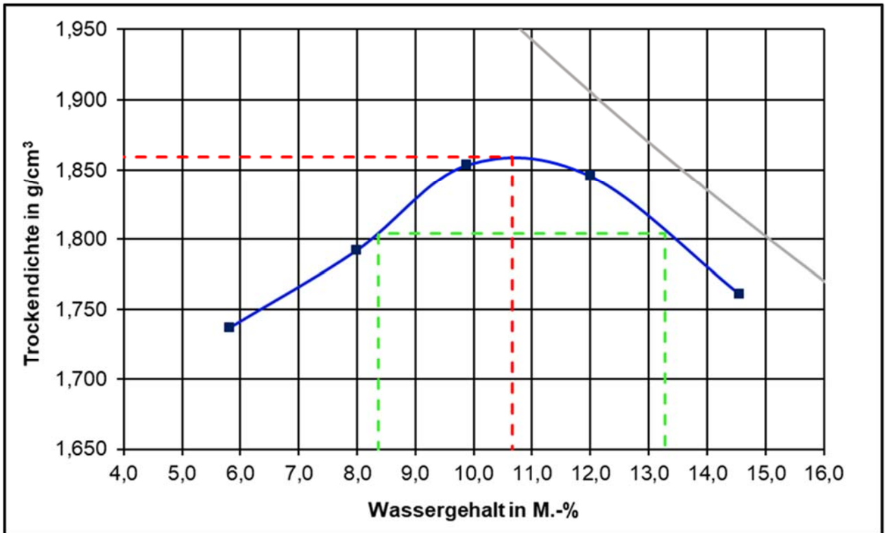
Proctorkurve des untersuchten RC-Materials 0/45 (aus Prüfbericht F 22/01/0043 – I/2022)
