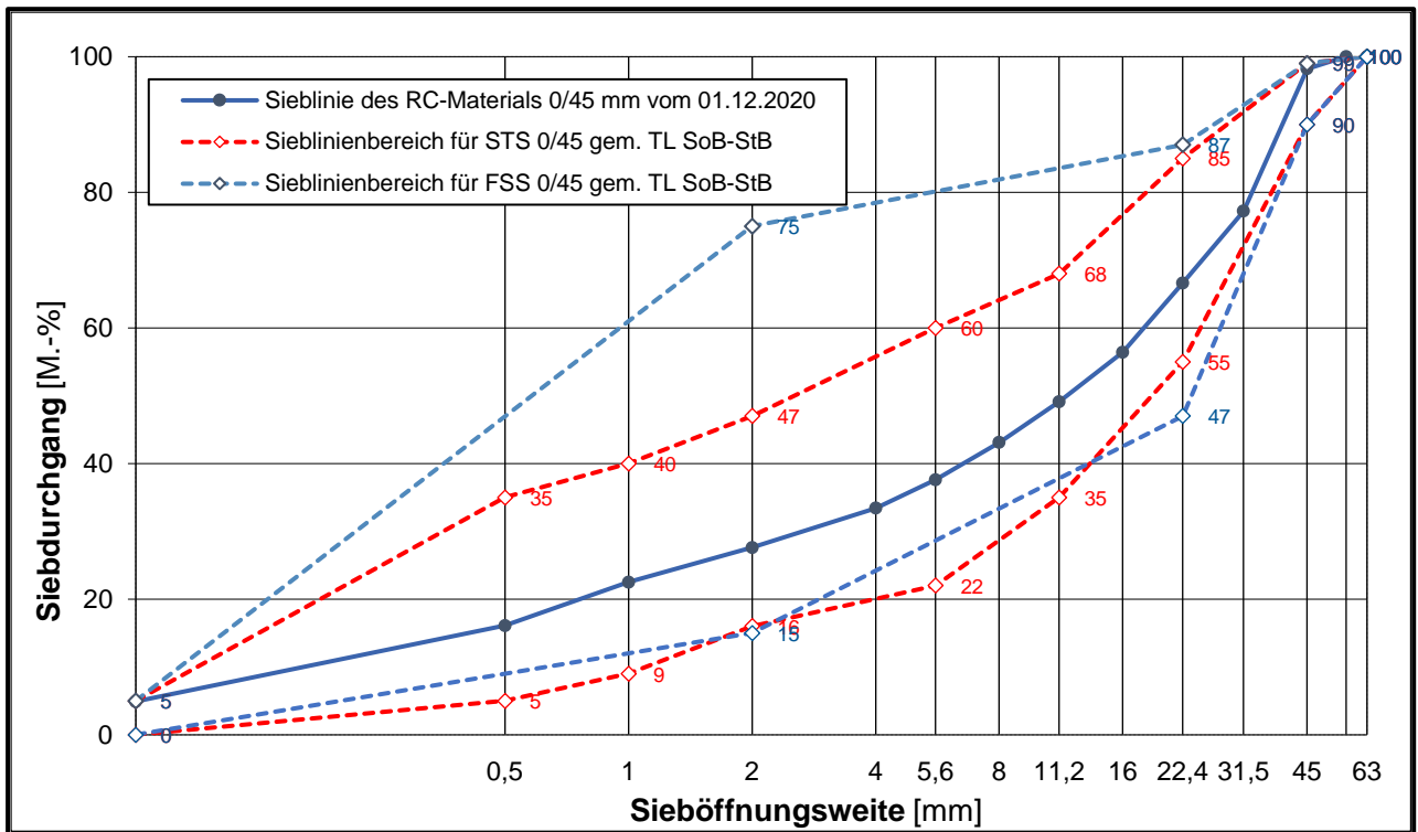
Korngrößenverteilung des untersuchten RC-Materials 0/45 mit Sieblinienbereich für Schottertragschichten 0/45 mm gemäß TL SoB-StB 7/7
