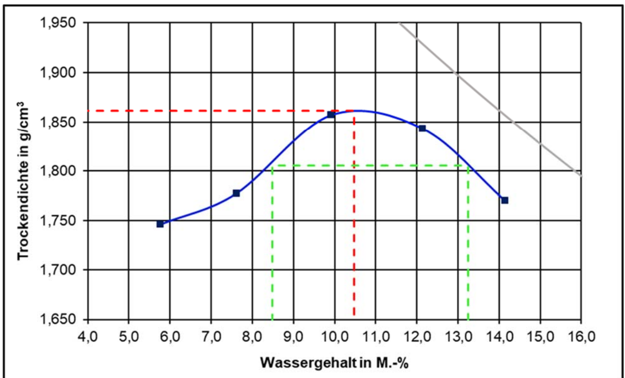
Proctorkurve des untersuchten RC-Materials 0/45 (aus Prüfbericht F 22/01/0056 – I/2022)
