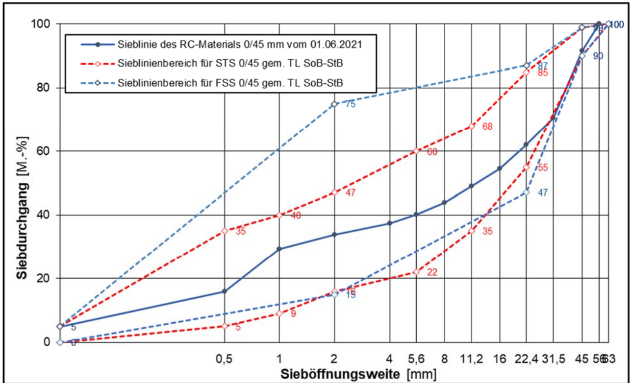
Korngrößenverteilung des untersuchten RC-Materials 0/45 mit Sieblinienbereich für Schottertragschichten 0/45 mm gemäß TL SoB-StB 7/
