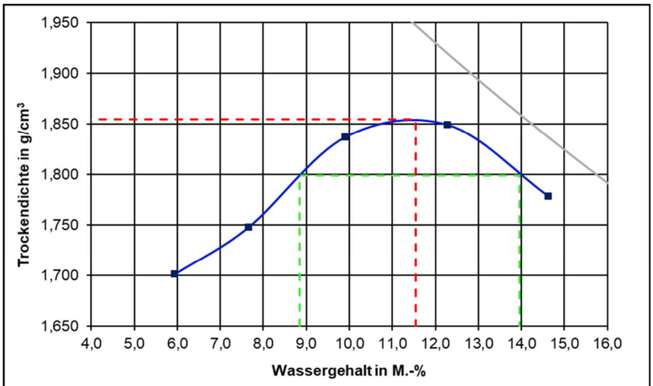
Proctorkurve des untersuchten RC-Materials 0/45
