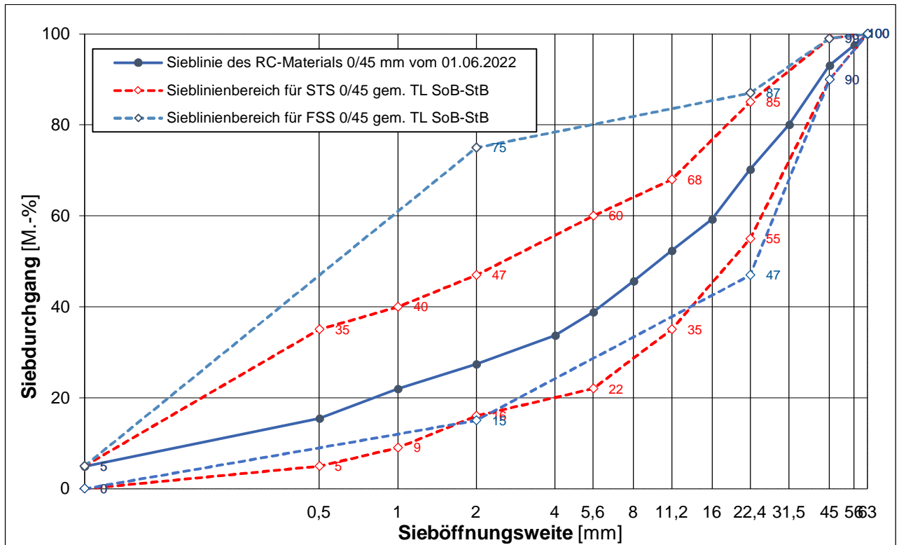
Korngrößenverteilung des untersuchten RC-Materials 0/45 mit Sieblinienbereich für Schottertrag- und Frostschutzschichten 0/45 mm gemäß TL SoB-StB /7/
