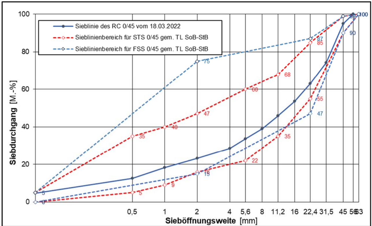
Korngrößenverteilung des untersuchten RC-Materials 0/45 mit Sieblinienbereich für Schottertragschichten 0/45 mm gemäß TL SoB-StB 7/7
