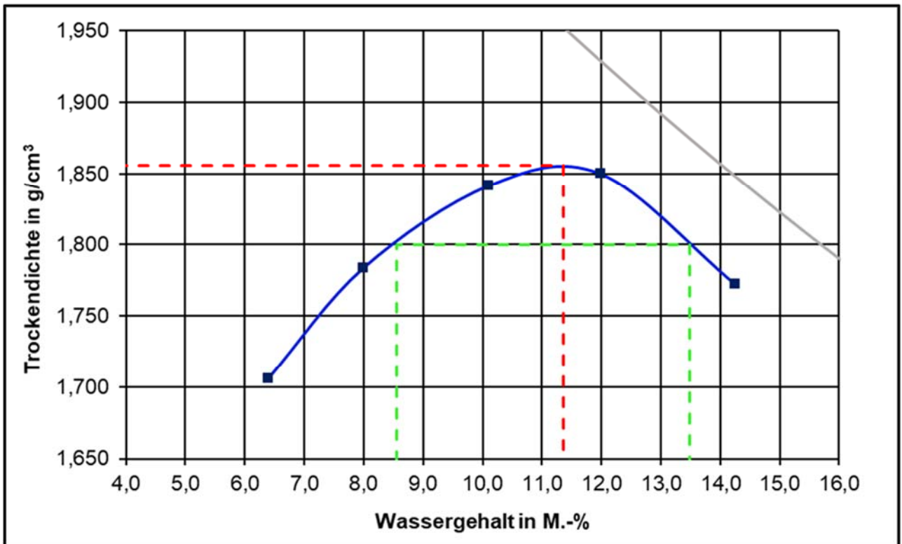
Proctorkurve des untersuchten RC-Materials 0/45 (aus Prüfbericht F 22/02/0123 – I/2022)
