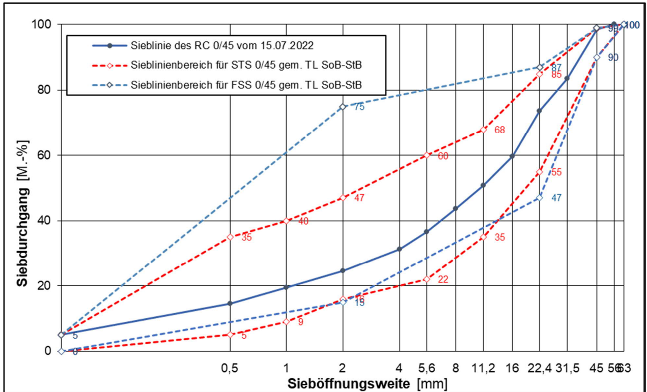
Korngrößenverteilung des untersuchten RC-Materials 0/45 mit Sieblinienbereich für Schottertrag- und Frostschutzschichten 0/45 mm gemäß TL SoB-StB //
