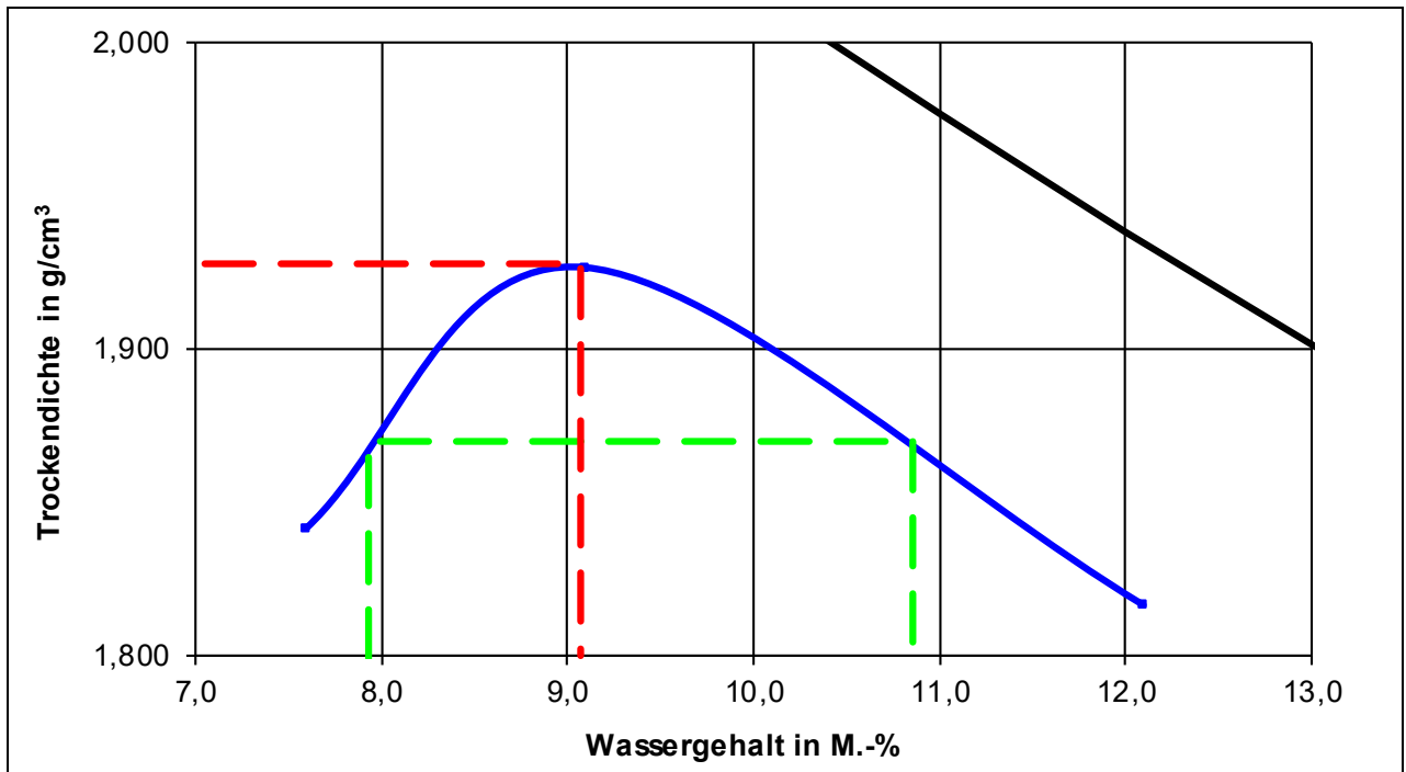
Proctorkurve des untersuchten RC-Materials 0/45 (aus Prüfbericht F 18/08/0718 – III/2018)
