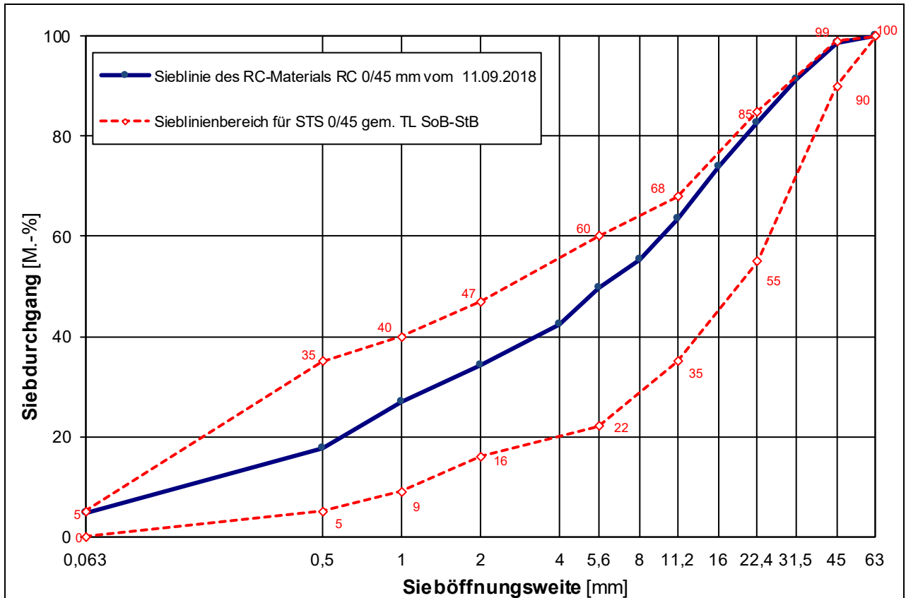
Korngrößenverteilung des untersuchten RC-Materials 0/45 mm mit Sieblinienbereich für Schottertragschichten 0/45 mm gemäß TL SoB-StB /7/
