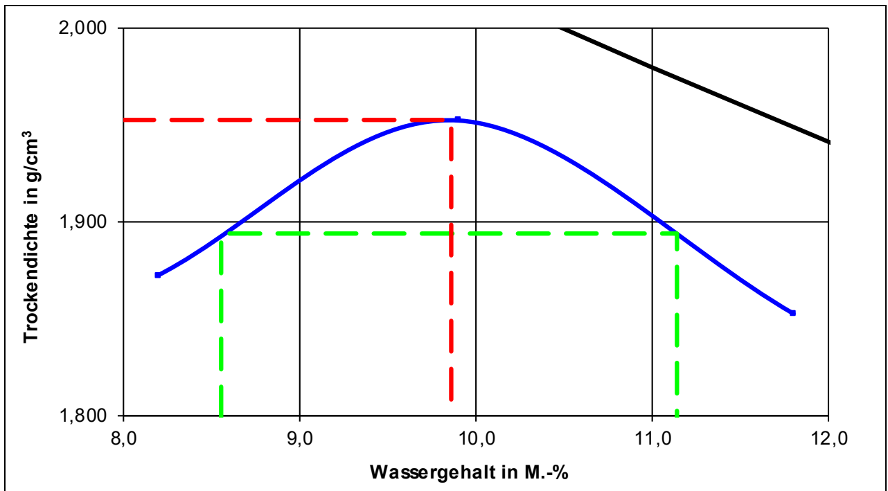
Proctorkurve des untersuchten RC-Materials 0/45 mm (aus Prüfbericht F 18/08/0711 – III/2018)
