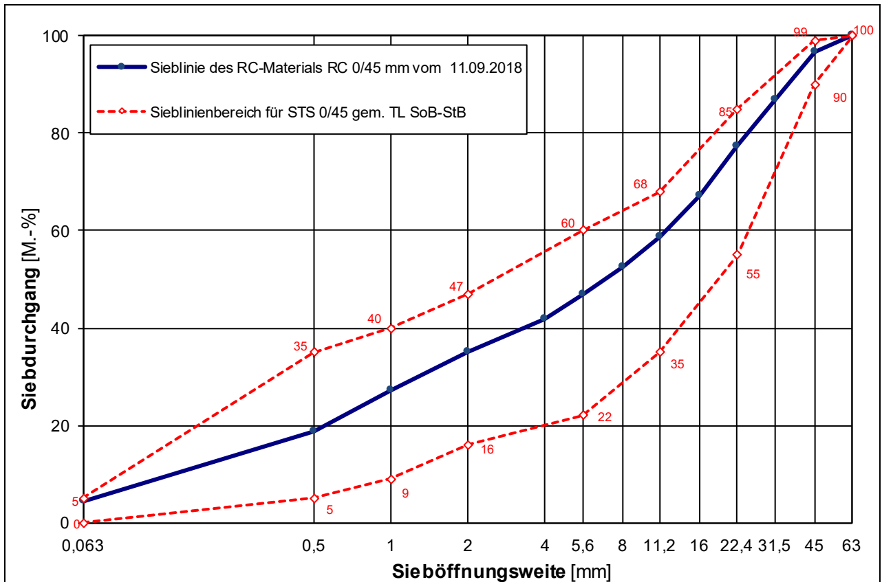
Korngrößenverteilung des untersuchten RC-Materials 0/45 mit Sieblinienbereich für Schottertragschichten 0/45 mm gemäß TL SoB-StB /7/
