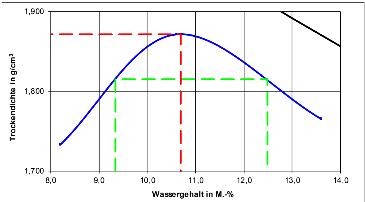
Proctorkurve des untersuchten RC-Materials 0/45 mm (aus Prüfbericht F 18/08/0712 – III/2018)
