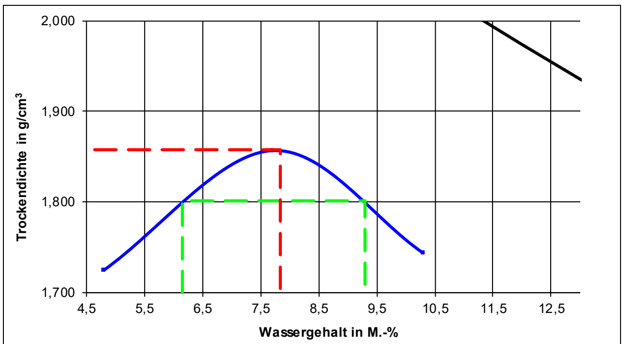
Proctorkurve des untersuchten RC-Materials 0/45 (aus Prüfbericht F 18/08/0714– III/2018)
